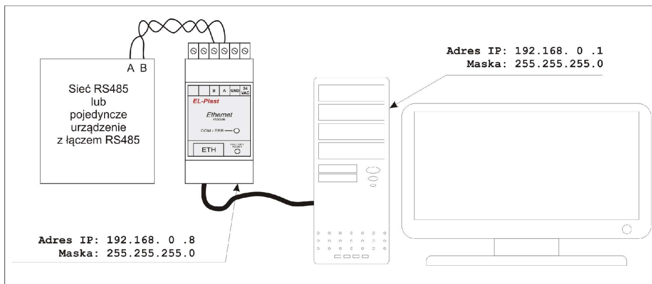
Podłączenie bezpośrednie
